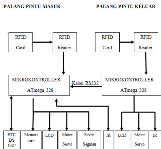
Gambar 7. Diagram Blok Sistem Parkir Otomatis
