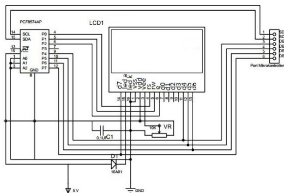
Gambar 3. Rangkaian LCD
