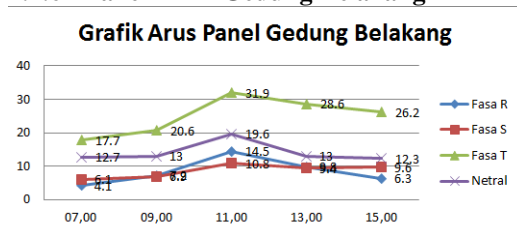
Gambar 9. Grafik arus panel mdp gedung belakang
