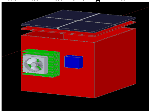
Gambar 7. Desain alat Pendingin Ikan
