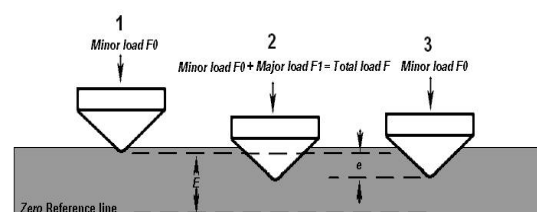
Gambar 2. Skema kondisi indenter
