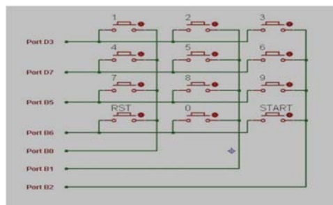
Gambar 4.1. Rangkaian Keypad
