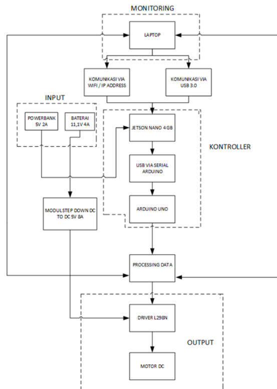
Gambar 1. Blok Diagram Sistem Kontroler Robot Mobil berbasis ROS
